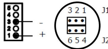
[20.3] Conexión con tensión externa. Colocar puente entre J1(2) y J2(5)
