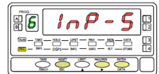
MENU 6 PROGRAMACIÓN DEL PIN 5
