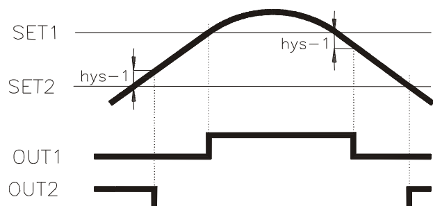
Actuación histéresis asimétrica
